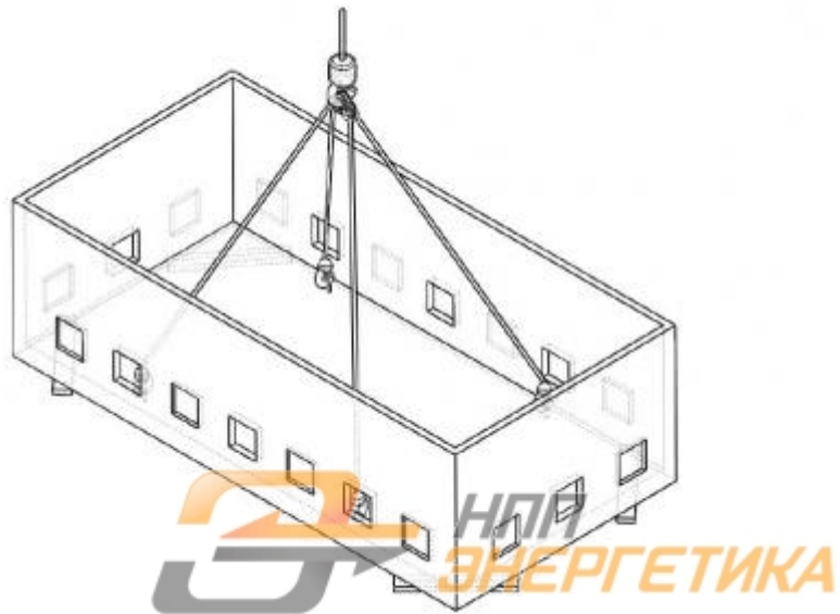
Схема складирования надземной и подземной части БК
